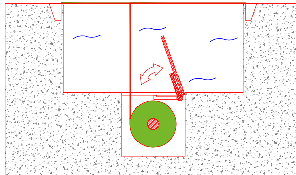
BEWEEGBARE KLEP 'VLINDER'
